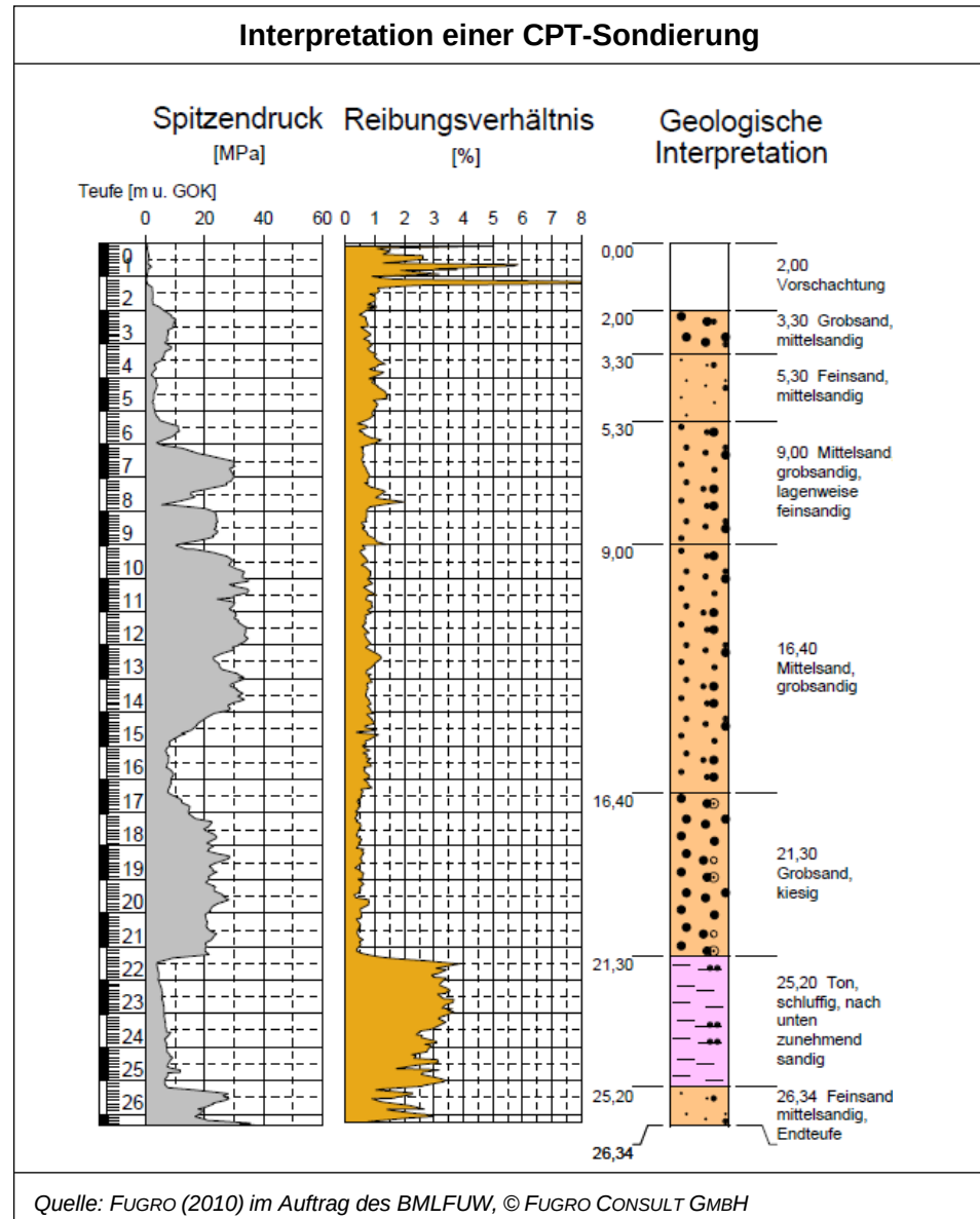
Abbildung 4: Interpretation einer CPT-Sondierung. Reibungsverhältnis = Verhältnis Mantelreibung/Spitzen- druck mal 100.
