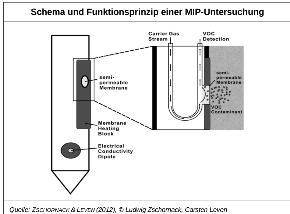
Abbildung 12: Schema und Funktionsprinzip einer MIP-Untersuchung.
