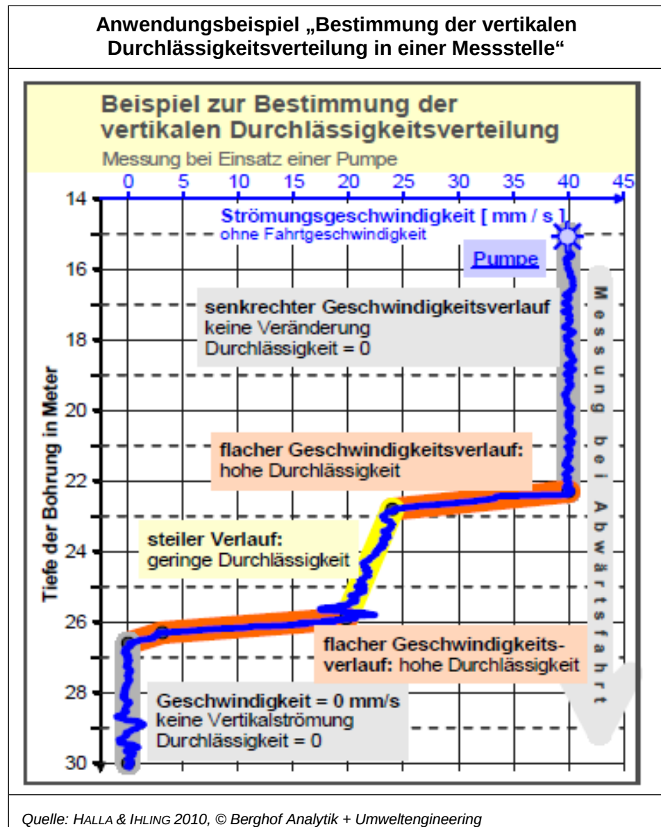
Abbildung 17: Anwendungsbeispiel „Bestimmung der vertikalen Durch- lässigkeitsverteilung in einer Messstelle“. In diesem Beispiel wurde das Flowmeter in der bepumpten Messstelle von oben nach unten geführt, die Ergebnisse sind bereits um die Fahrtgeschwindigkeit der Sonde bereinigt.
