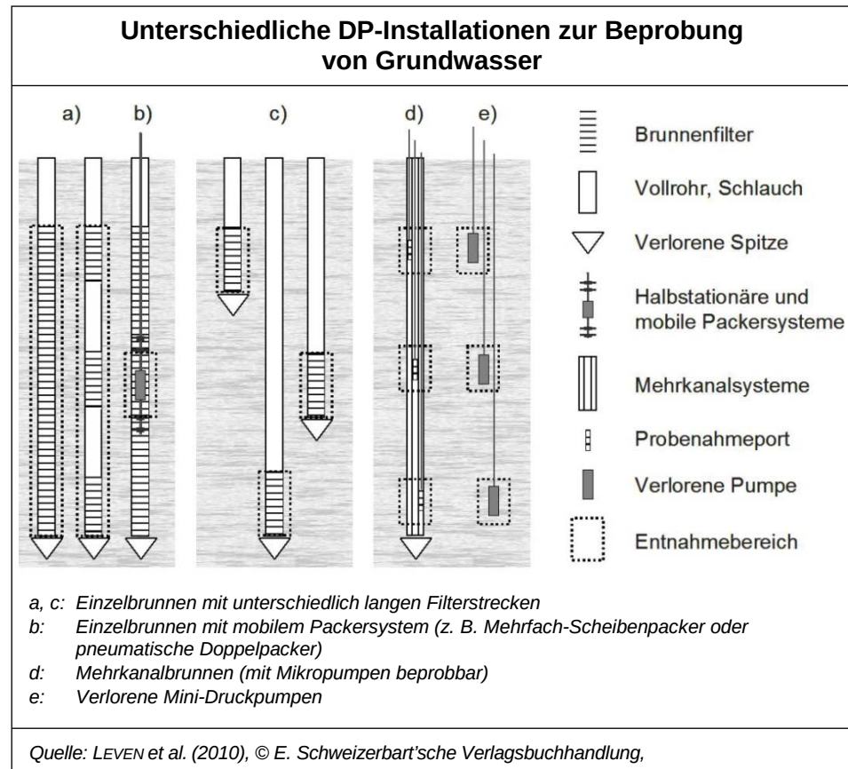
Abbildung 10: Unterschiedliche DP- Installationen zur Beprobung von Grundwasser.
