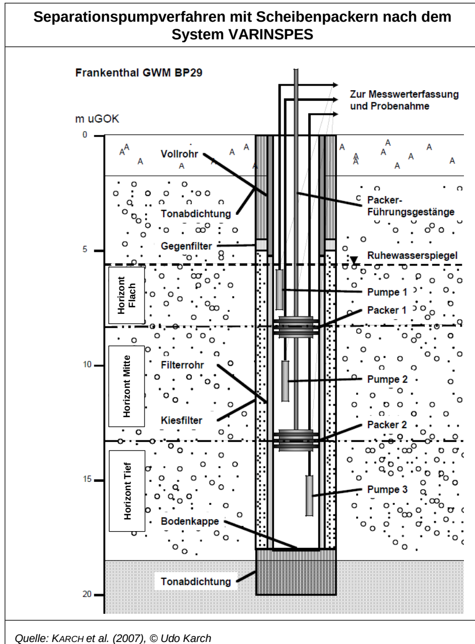
Abbildung 23: Separationspump- verfahren mit Scheibenpackern nach dem System VARINSPES.
