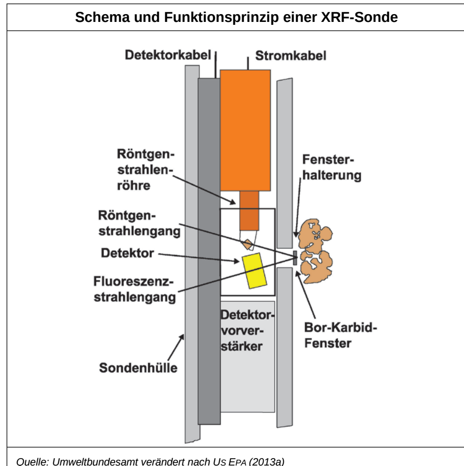
Abbildung 16: Schema und Funktionsprinzip einer XRF-Sonde.
