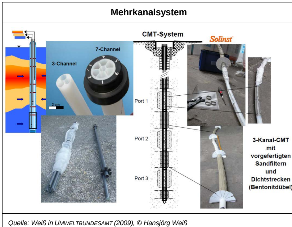
Abbildung 11: Mehrkanalsystem (CMT: Continuous Multi- Channel Tubing) zur gleichzeitigen Beprobung unterschiedlicher Tiefenhorizonte im Grundwasser.
