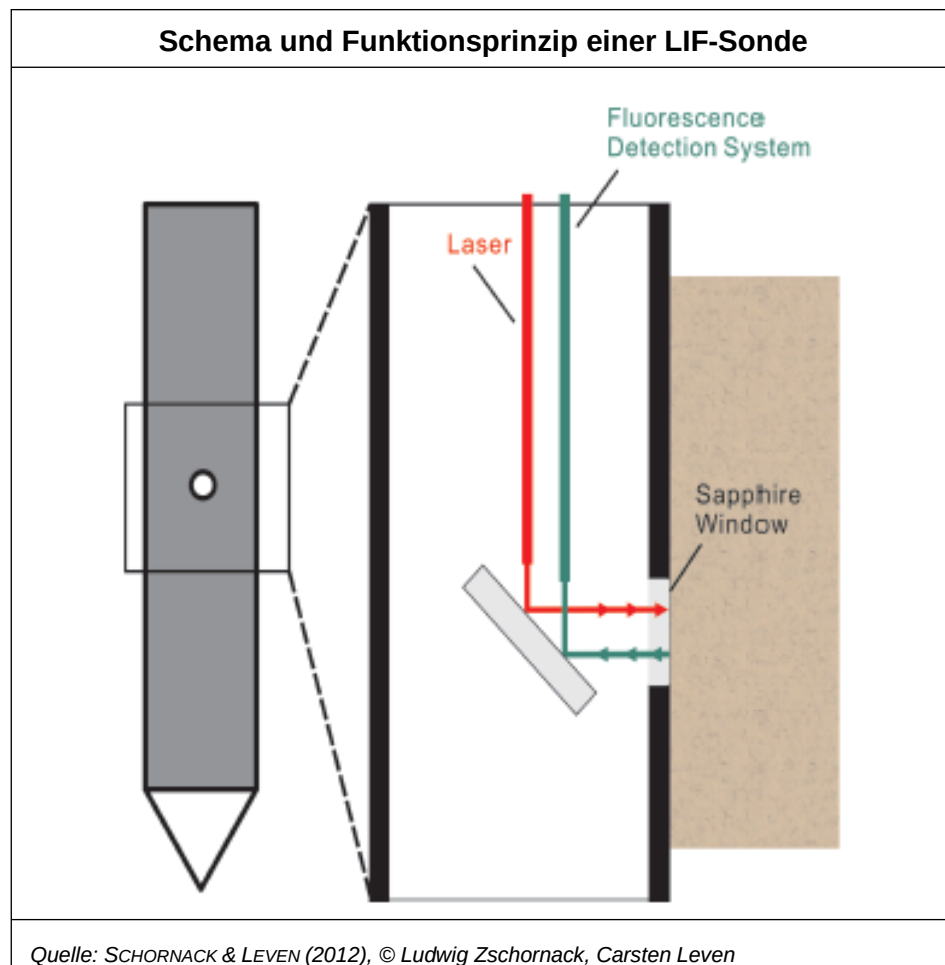
Abbildung 14: Schema und Funktionsprinzip einer LIF-Sonde.
