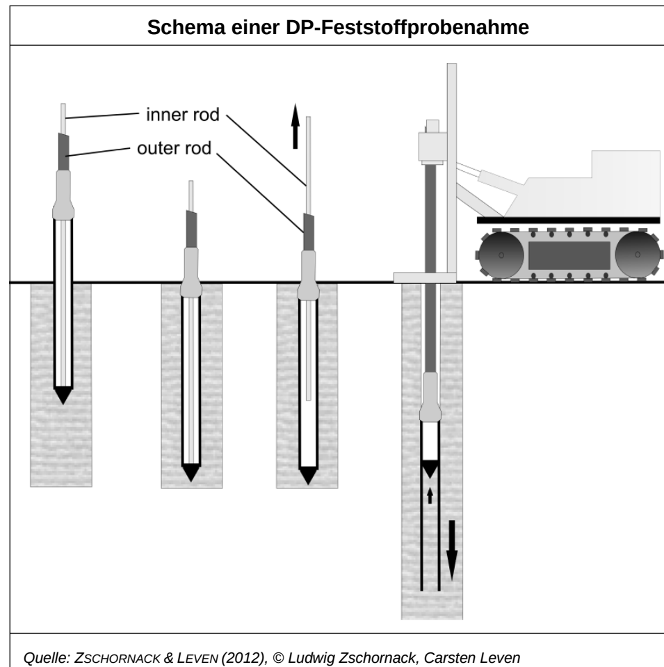
Abbildung 7: Schema einer DP- Feststoffprobenahme (Einzelprobe) mit ziehbarem Innengestänge.
