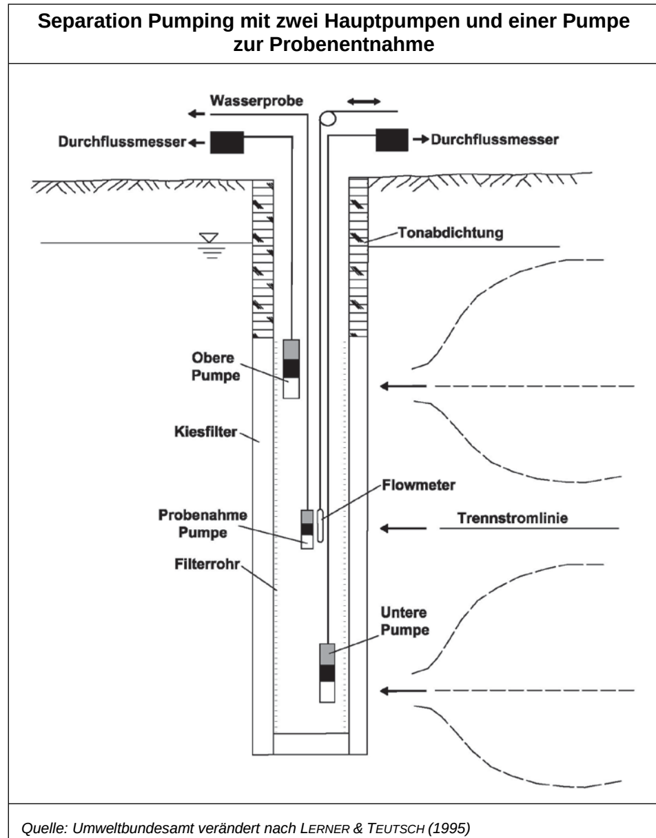
Abbildung 22: Separation Pumping mit zwei Hauptpumpen und einer Pumpe zur Probenentnahme.
