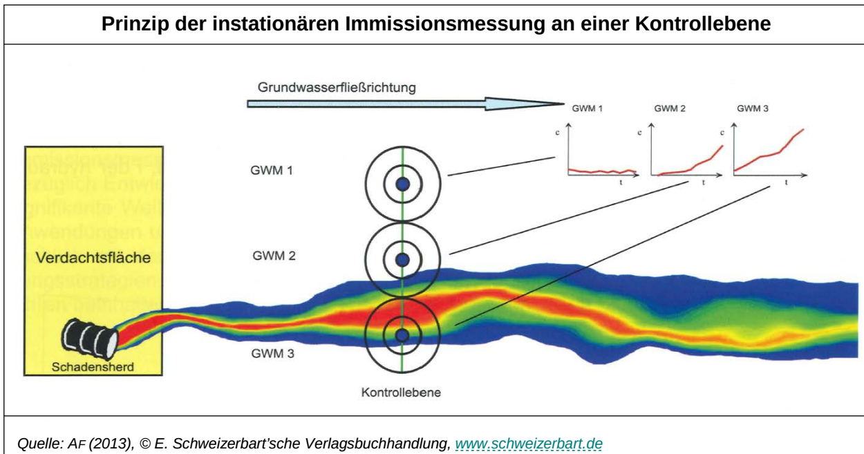
Abbildung 21: Prinzip der instationären Immissionsmessung an einer Kontrollebene.
