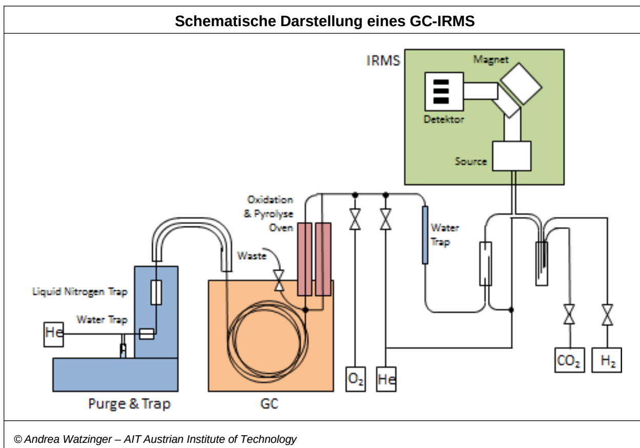
Abbildung 40: Schematische Darstellung eines GC-IRMS.
