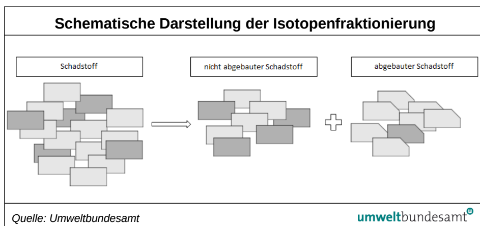
Abbildung 39: Schematische Darstellung der Isotopenfraktionierung durch mikrobiellen Abbau, hellgrau: Moleküle ohne ^{13}\text{C} , dunkelgrau: Moleküle mit ^{13}\text{C} .
