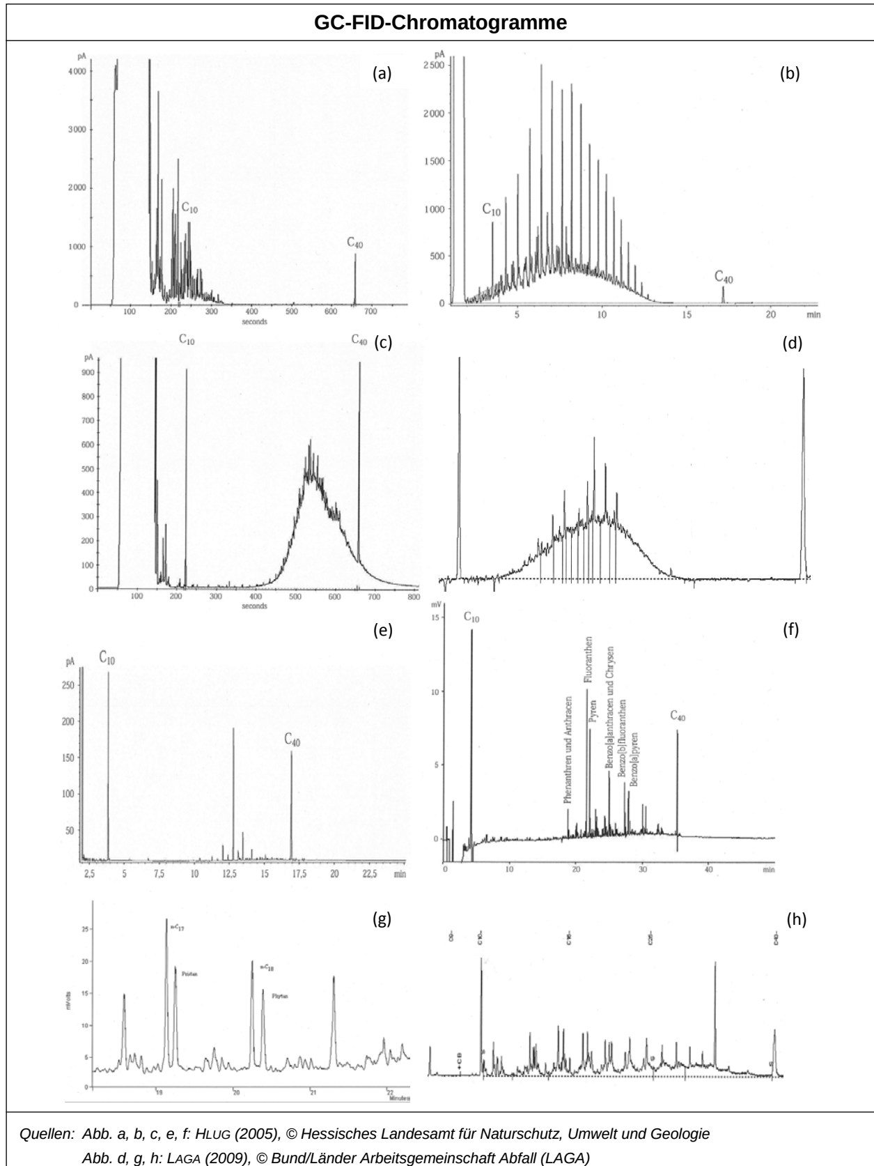
(a) Superplus-Benzin, (b) Diesel, (c) Motoröl, (d) gealterter Dieselschaden, (e) Waldboden, humushaltig, (f) Boden, PAK-haltig, (g) Peaks von n\text{-C}_{17} , Pristan, n\text{-C}_{18} , Phytan, (h) Polypropylen, homologe Iso- und Cycloalkan und Alken-Verteilung
