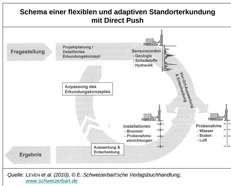
Abbildung 2: Schema einer flexiblen und adaptiven Standorterkundung mit Direct Push.
