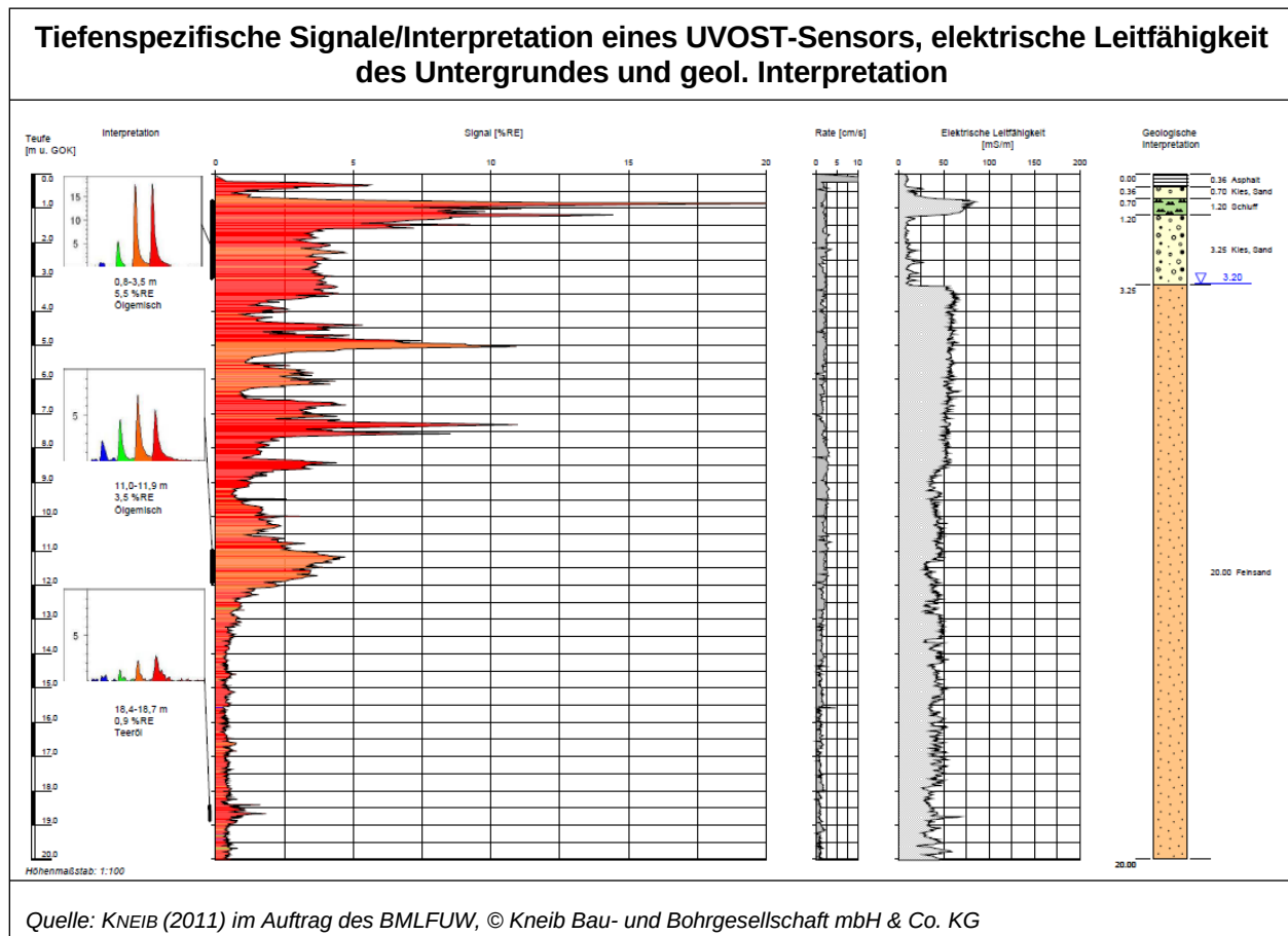
Abbildung 15: Tiefenspezifische Signale/Interpretation eines UVOST-Sensors, elektrische Leitfähigkeit des Untergrundes und geol. Interpretation.
