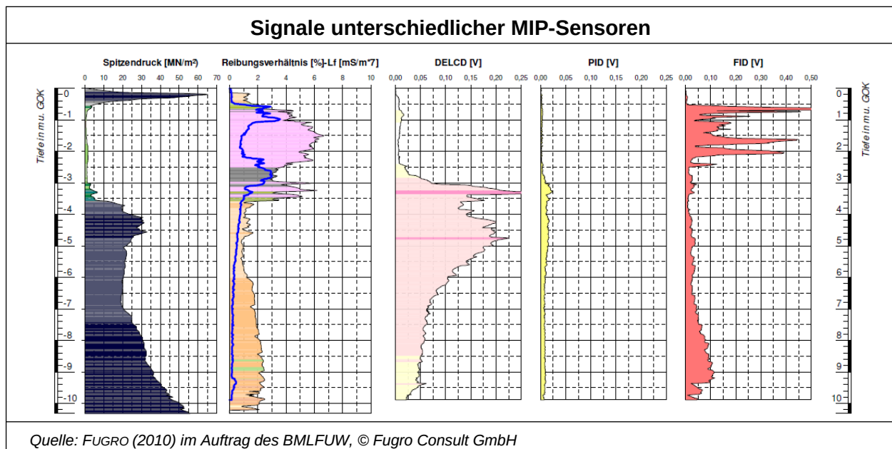
Abbildung 13: Signale unterschiedlicher MIP-Sensoren (DELCD, PID, FID), elektrische Leitfähigkeit des Untergrundes (blaue Linie) und Ergebnisse einer CPT-Untersuchung (Spitzendruck und Reibungsverhältnis).
