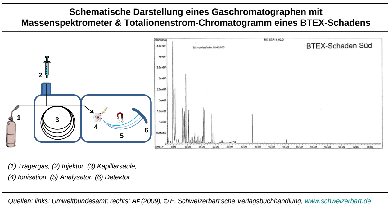
Abbildung 37: links: schematische Darstellung eines Gaschromatographen mit Massenspektrometer rechts: Totalionenstrom-Chromatogramm eines BTEX-Schadens.
