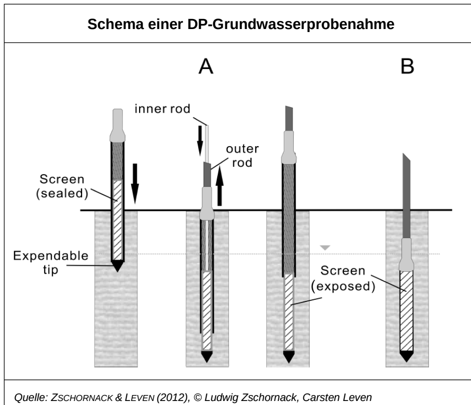
Abbildung 8: Schema einer DP-Grundwasserprobenahme mit geschütztem (A) und ungeschütztem (B) Filterelement.
