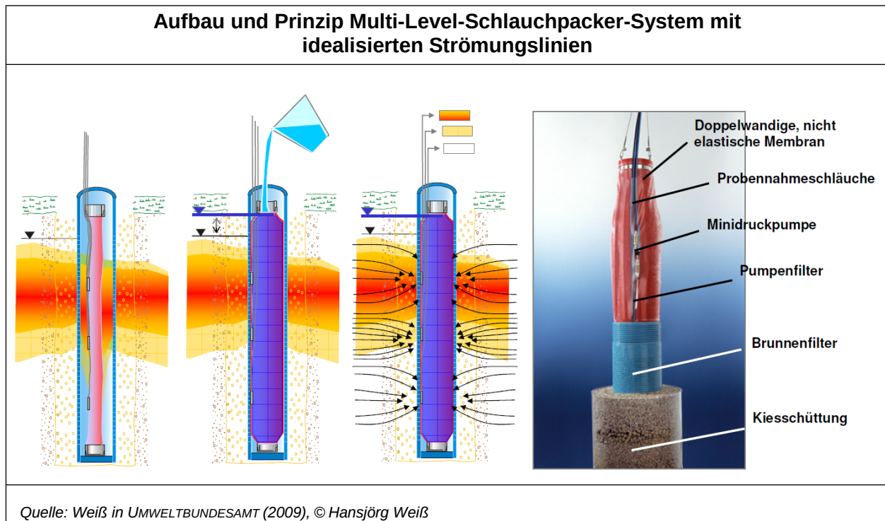
Abbildung 24: Aufbau und Prinzip Multi-Level-Schlauchpacker-System mit idealisierten Strömungslinien.
