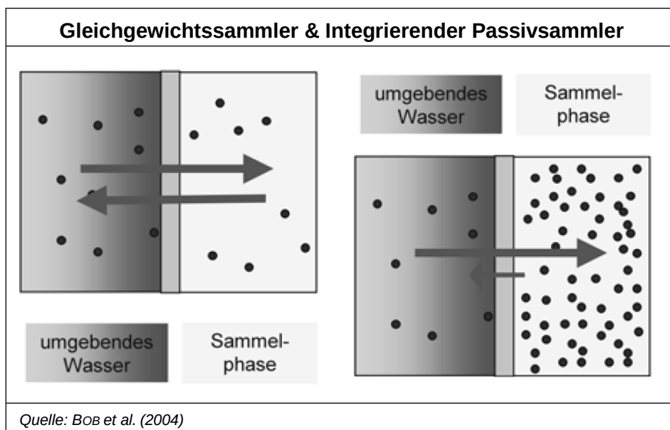
Abbildung 26: links: Gleichgewichtssammler – das Konzentrationsgleichgewicht zwischen Sammelmedium und umgebendem Wasser wird ausgeglichen. Es findet keine Schadstoffaufkonzentration statt. rechts: Integrierender Passivsammler – die Aufnahmekapazität des Sammelmediums darf im Expositionszeitraum nicht erreicht werden.
