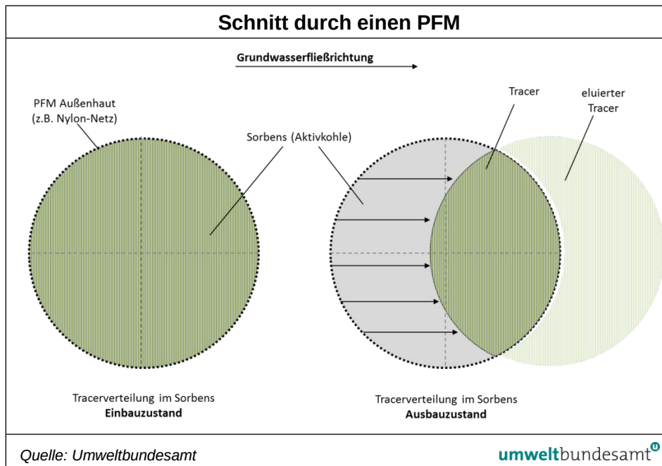
Abbildung 30: Schnitt durch einen PFM (links Einbauzustand, rechts Ausbauzustand).
