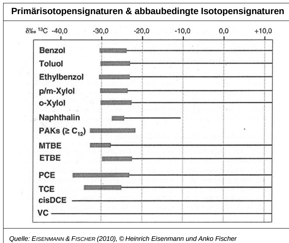
Abbildung 41: Primärisotopen- signaturen (Balken) und abbaubedingte Isotopensignaturen (Linien) für häufige Schadstoffe.
