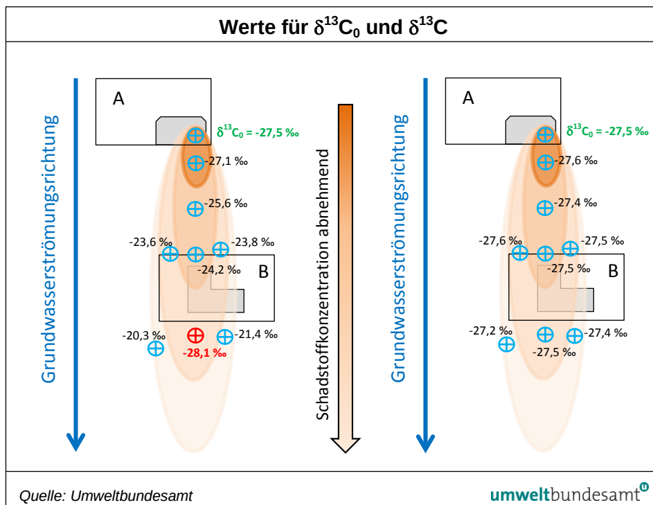
Abbildung 42: Werte für \delta^{13}\text{C}_0 und \delta^{13}\text{C} .
