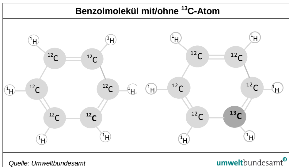
Abbildung 38: links: Benzolmolekül mit ausschließlich ^{12}\text{C} -Atomen (rd. 94 %) rechts: Benzolmolekül mit einem ^{13}\text{C} -Atom (rd. 6 %).
