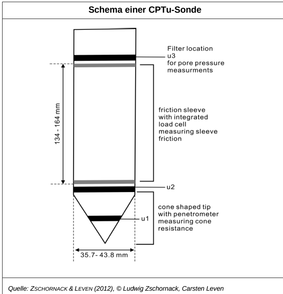
Abbildung 3: Schema einer CPTu- Sonde.
