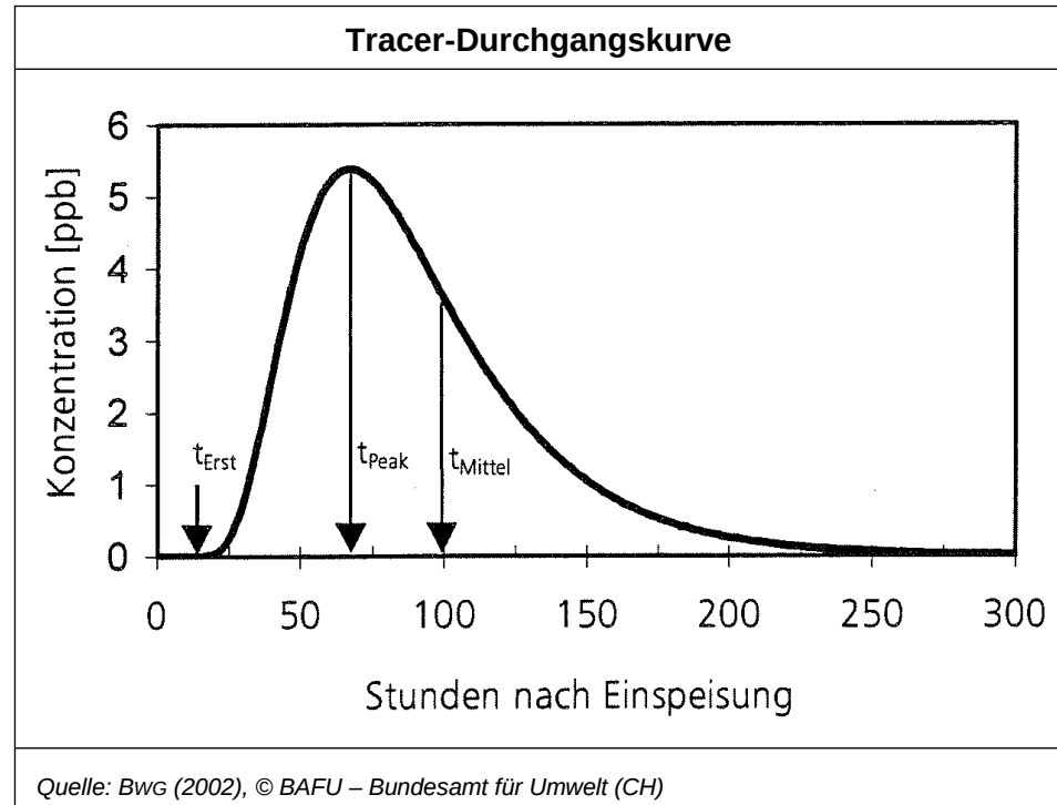
Abbildung 32: Tracer-Durchgangskurve; Erstaufreten = minimale Fließzeit ( t_{\text{Erst}} ), Maximum = Peak-Fließzeit ( t_{\text{Peak}} ), mittlere Fließzeit ( t_{\text{Mittel}} ).
