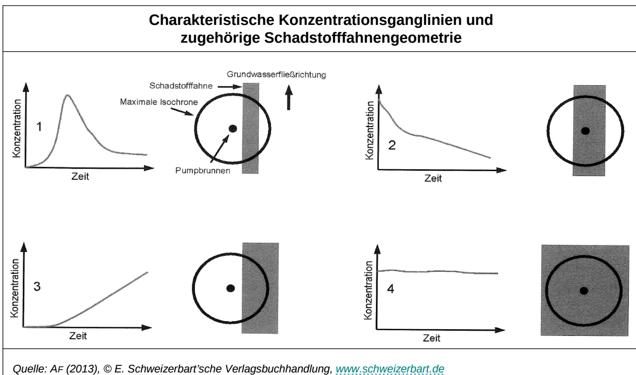
Abbildung 20: Charakteristische Konzentrationsganglinien und zugehörige Schadstofffahnengeometrie.
