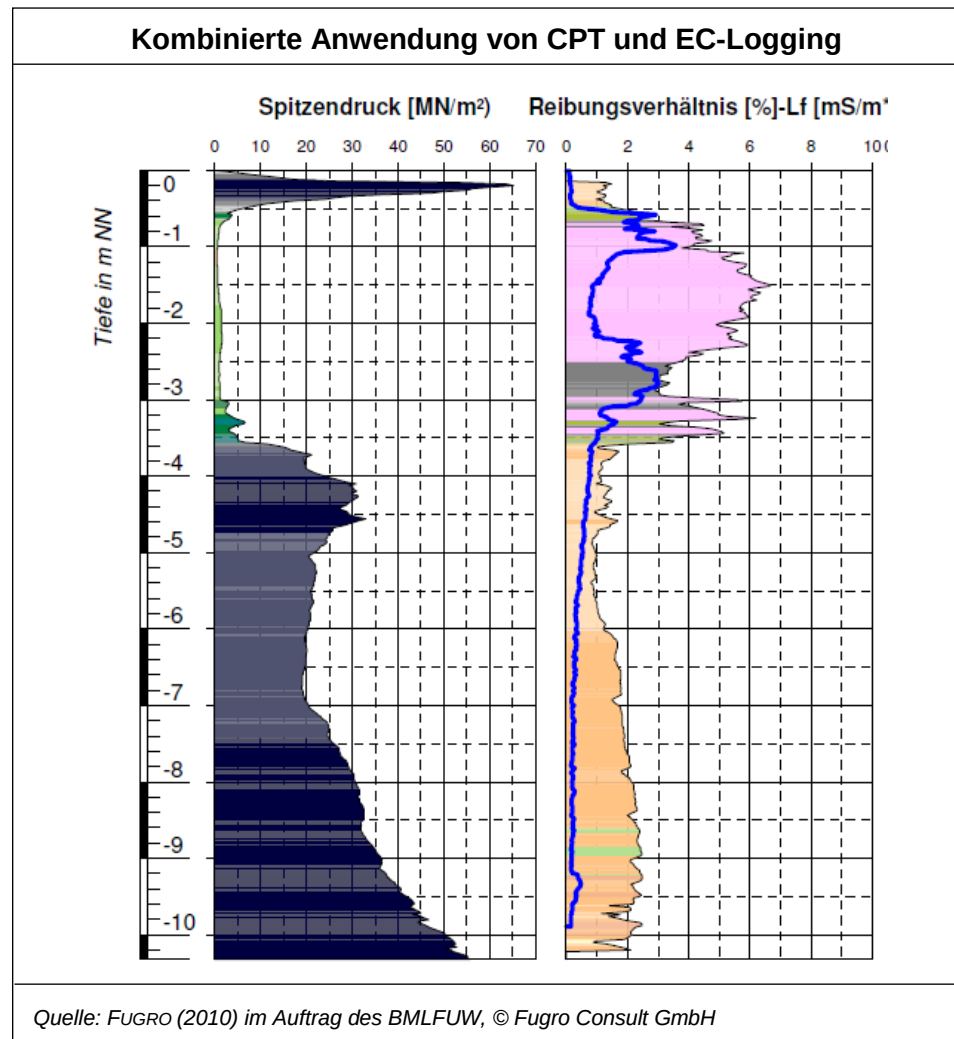
Abbildung 6: Kombinierte Anwendung von CPT und EC- Logging (blaue Linie).
