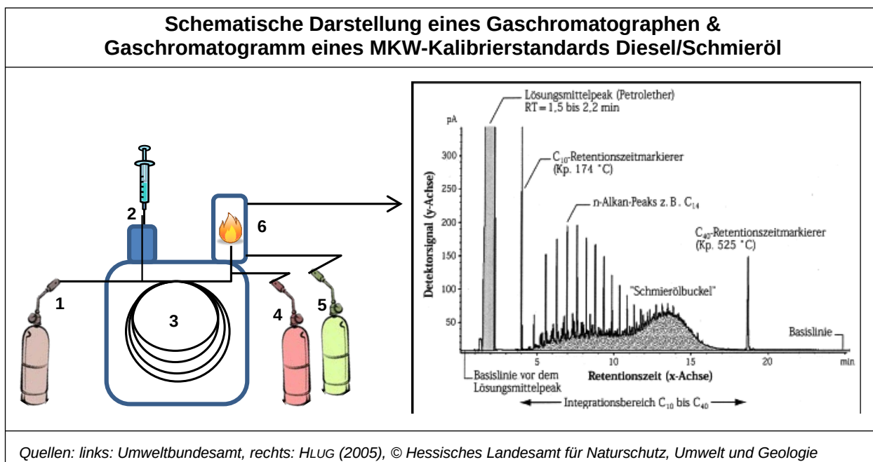
Abbildung 35: links: schematische Darstellung eines Gaschromatographen mit Flammenionisationsdetektor: (1) Trägergas, (2) Injektor, (3) Kapillarsäule, (4) Wasserstoff, (5) Luft, (6) FID rechts: Gaschromatogramm eines MKW-Kalibrierstandards Diesel/Schmieröl.
