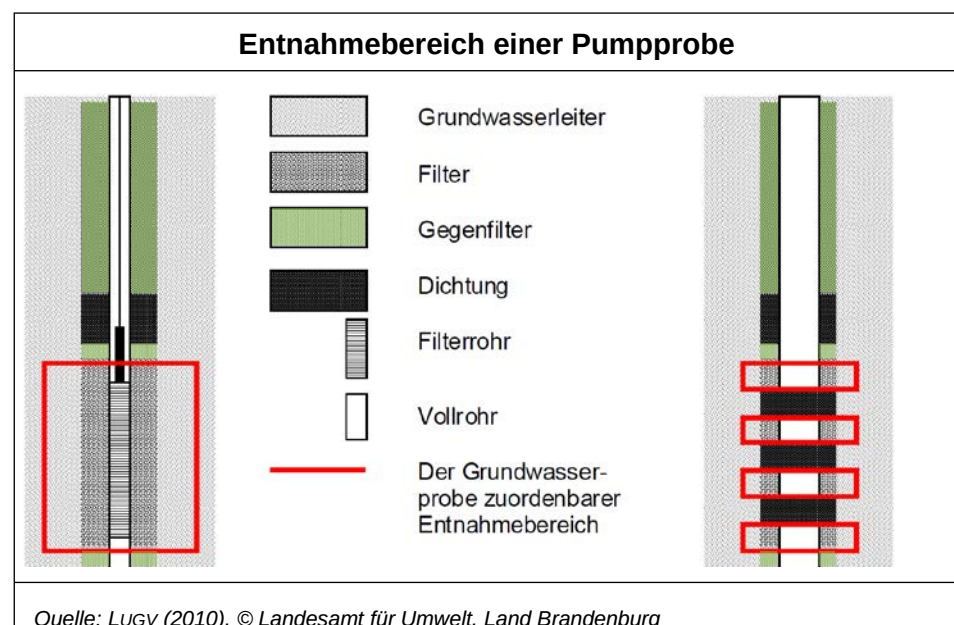
Abbildung 25: Entnahmebereich einer Pumpprobe aus einer voll-verfilterten, konventionellen Messstelle (links) im Vergleich zu einer tiefenorientiert ausge- bauten Sondermess- stelle (Multiproben- nahme-System) bei geringen Entnahmeraten (rechts).
