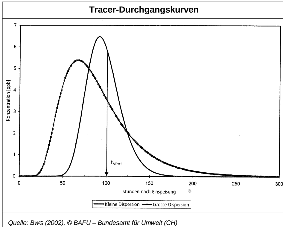
Abbildung 33: Tracer-Durchgangs- kurven mit gleicher mittlerer Fließzeit t_{\text{Mittel}} jedoch unterschiedlichen Dispersionskoeffizienten und Fließzeiten t_{\text{Erst}} und t_{\text{Peak}} .
